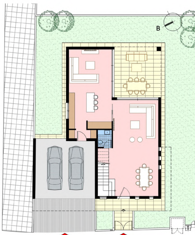
ΚΑΤΟΨΗ ΙΣΟΓΕΙΟΥ
