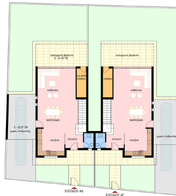
ΚΑΤΟΨΗ ΙΣΟΓΕΙΟΥ
