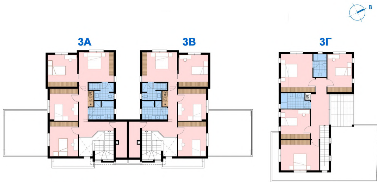
ΚΑΤΟΨΗ ΟΡΟΦΗΣ
