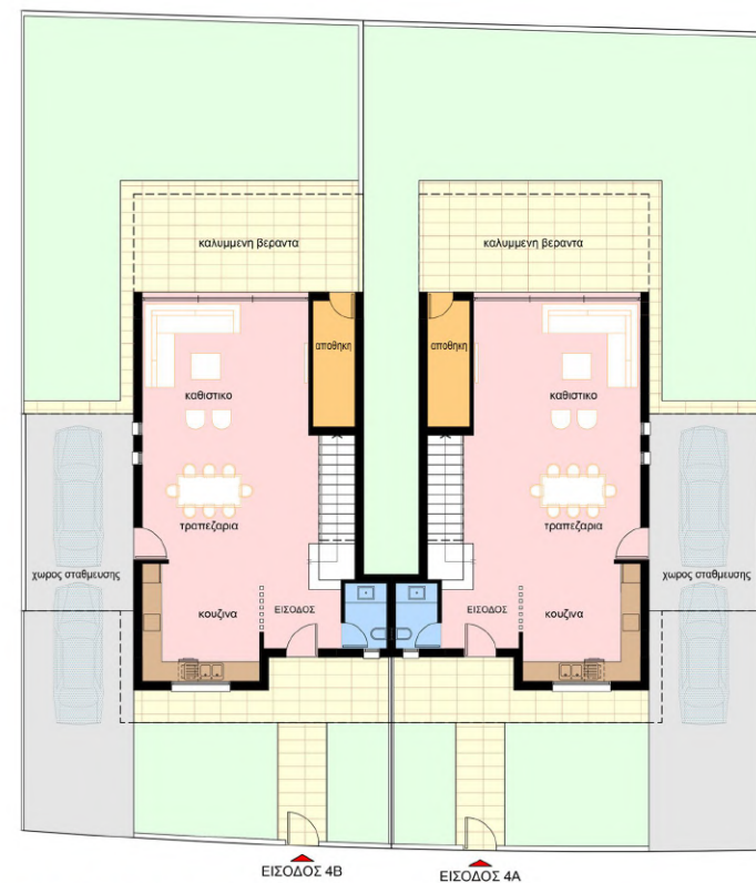
ΚΑΤΩΗ ΙΣΟΓΕΙΟΥ
